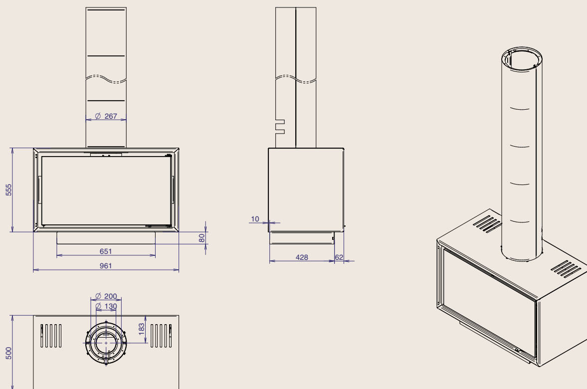
schéma Vénus True Vision C850 Caisson simple face Buse décorative en option
