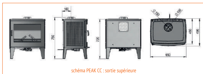
schéma PEAK CC : sortie supérieure
