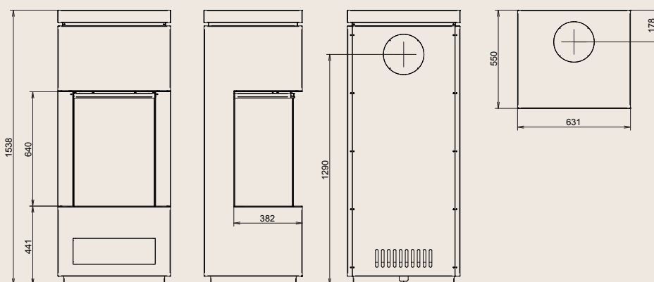
schéma Poêle True Vision 550 PDC
